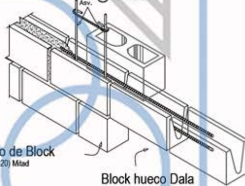
Grapa @ 2 hiladas
